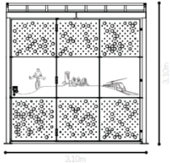
Alzado frontal
