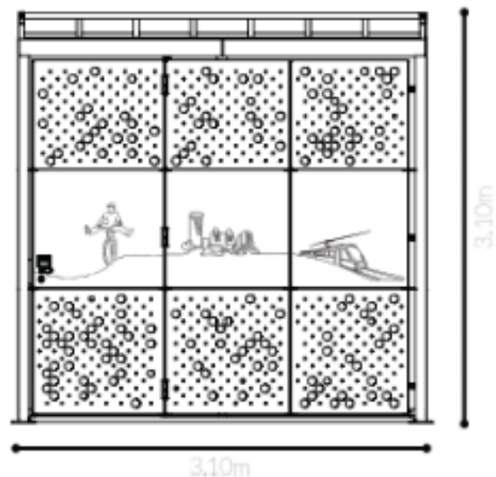
Alzado frontal
